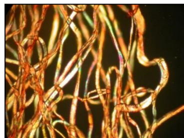
شکل ۲: تصویر میکروسکوپی نمونه‌ی شماره یک با نور پلاریزان و شناسایی لیف پنبه
